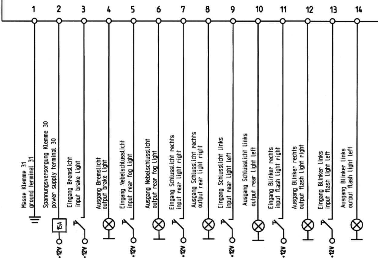
14 polige Steckerleiste des Moduls 321212 14 pin connector of 321212 control module
