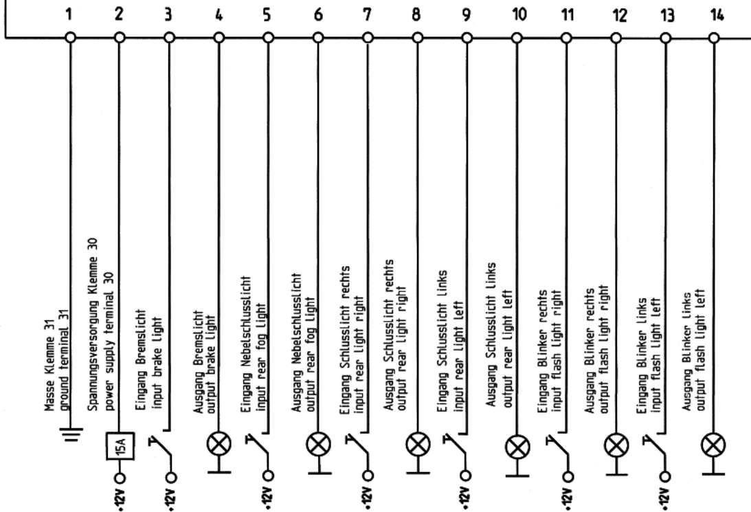
14 polige Steckerleiste des Moduls 321117 14 pin connector of 321117 control module
